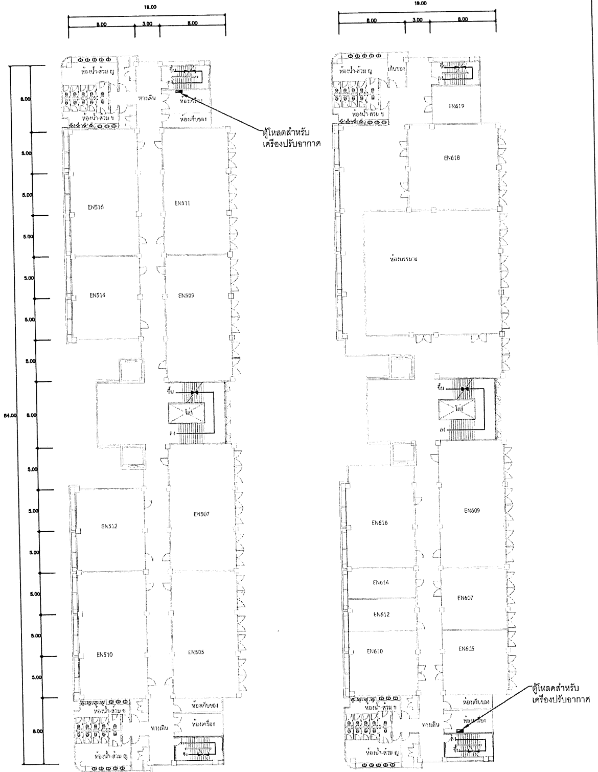
แปลน ชั้นที่ 6
