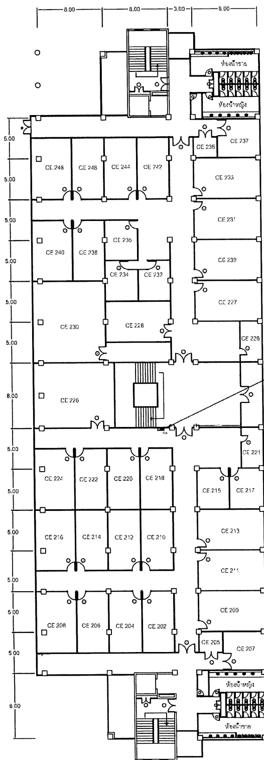
แปลน ชั้นที่ 2
