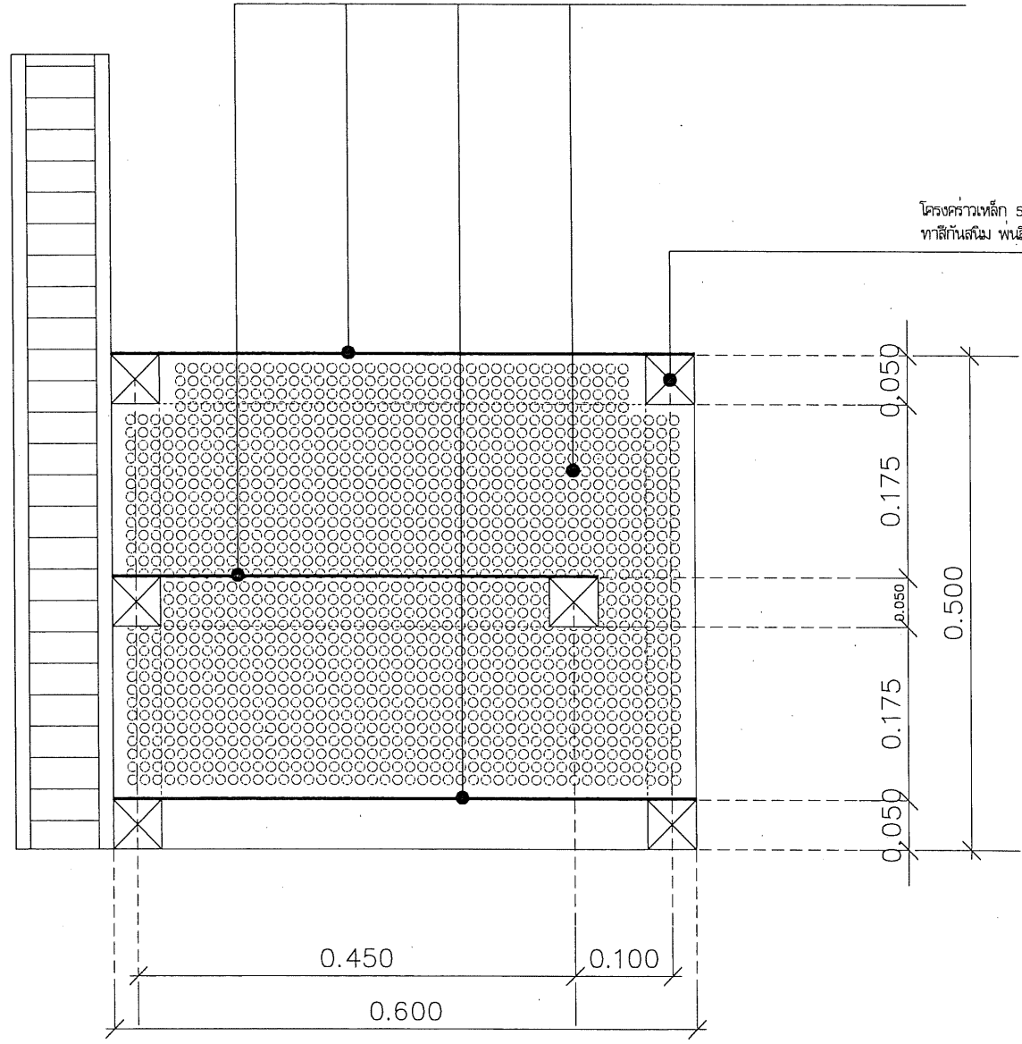
รูปตัด A มาตราส่วน No Scale
